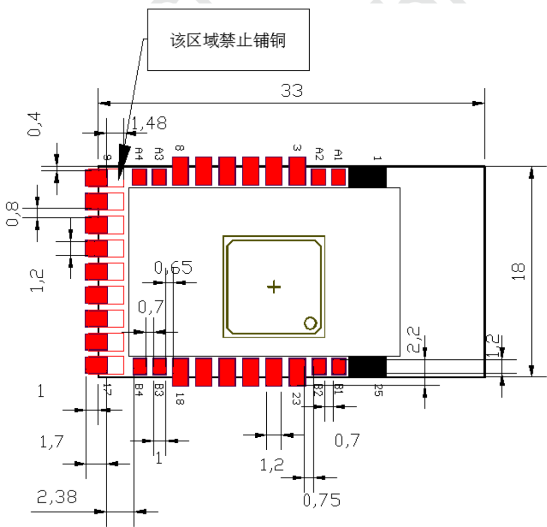
图 4 邮票孔封装尺寸图
